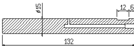
G3/052 perno/pin
